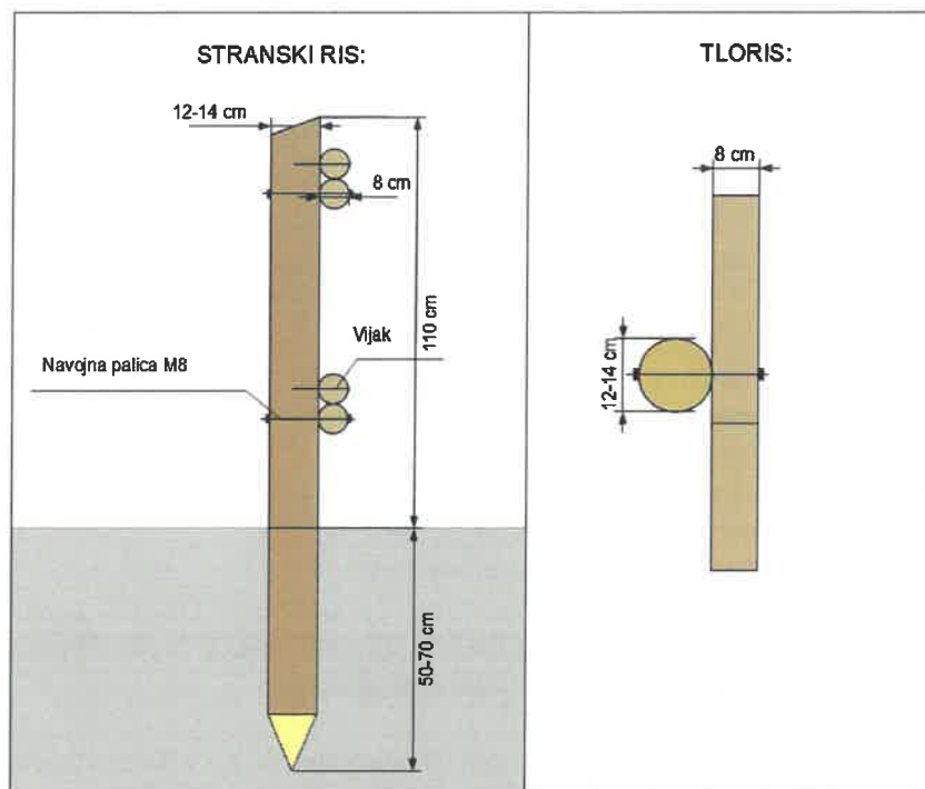
Slika 2: Stranski ris in tloris izvedbe lesene pašne ograje
