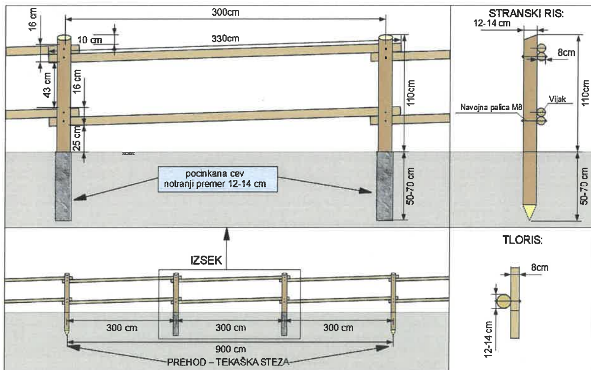
Slika 3: Značilni prerezi izvedbe lesene pašne ograje na mestu prehoda čez tekaško stezo (prehod 1)
