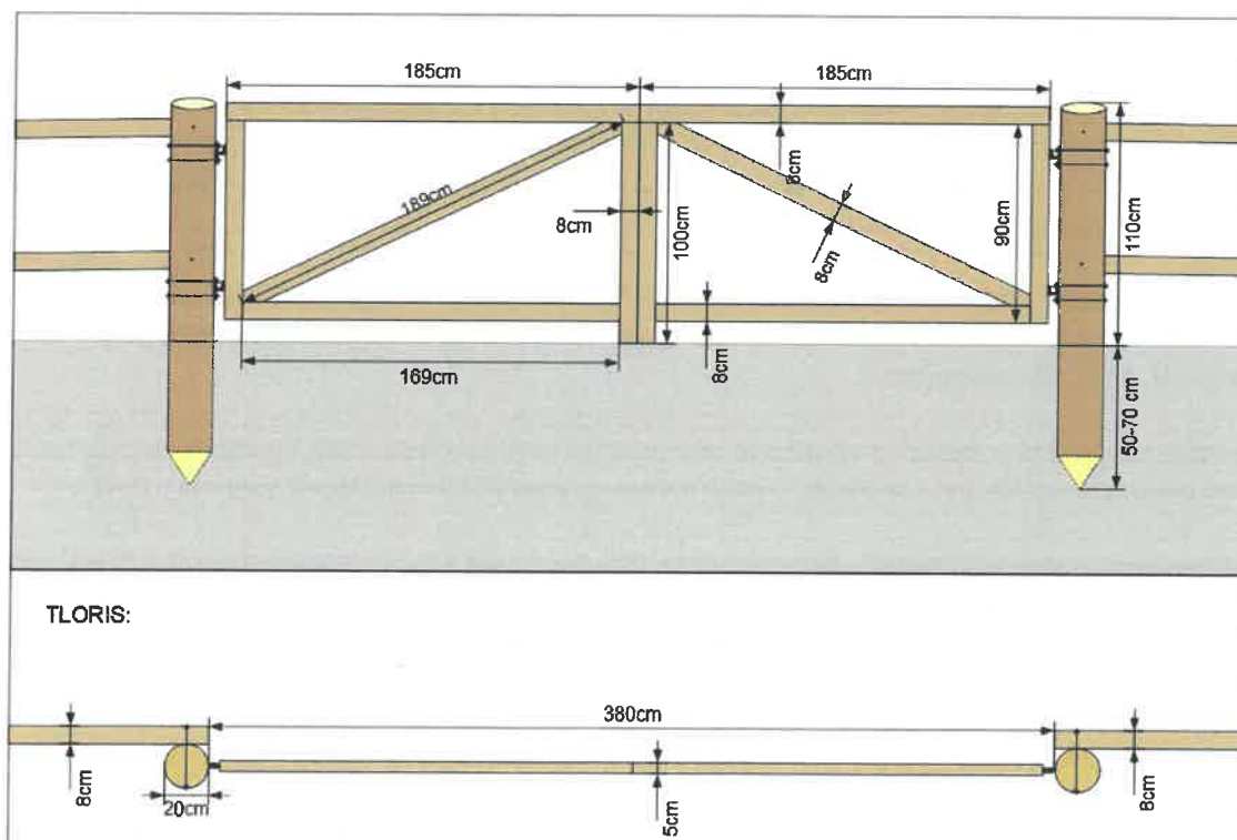
Slika 4: Značilni prerezi izvedbe lesene pašne ograje na mestu prehoda za učno pot (prehod 2)
