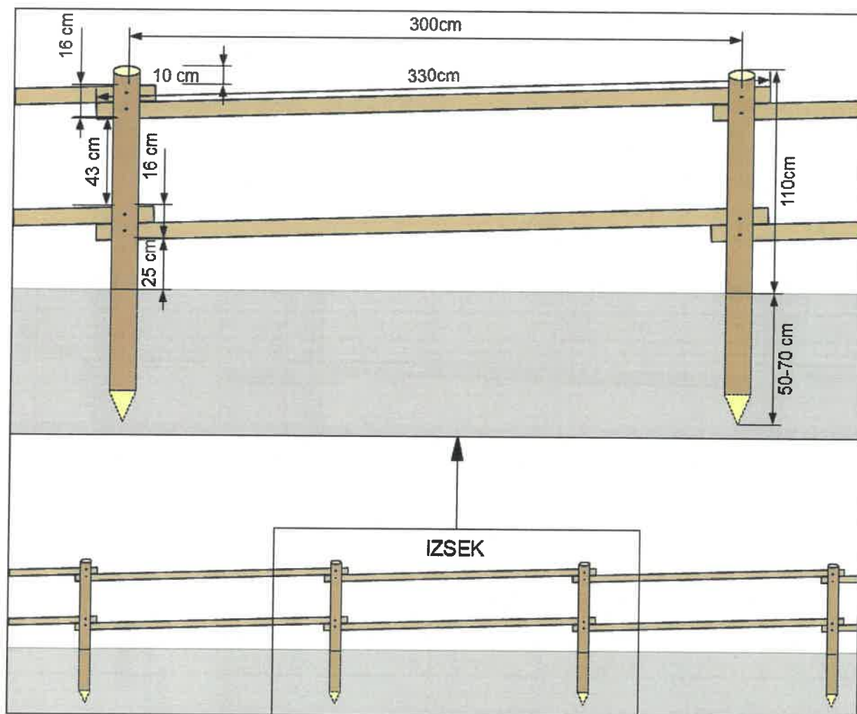
Slika 1: Značilen prerez izvedbe lesene pašne ograje
