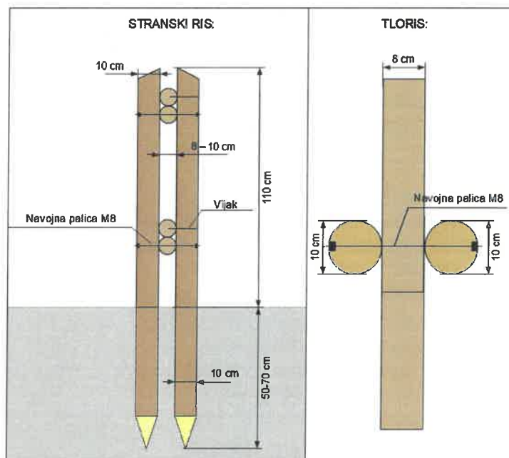
Slika 2: Stranski ris in tloris izvedbe lesene pašne ograje
