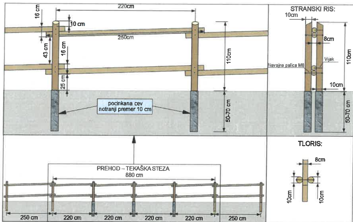
Slika 3: Značilni prerezi izvedbe lesene pašne ograje na mestu prehoda čez tekaško stezo
