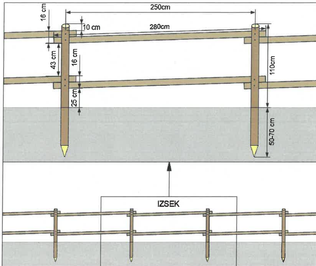
Slika 1: Značilen prerez izvedbe lesene pašne ograje
